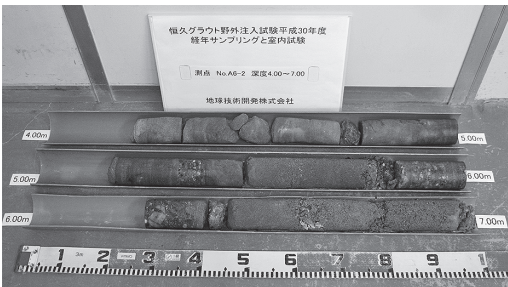
写真3 ハイブリッドシリカ(経年19年)
