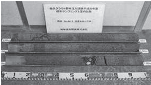
写真4 シリカゾルグラウト(経年19年)
